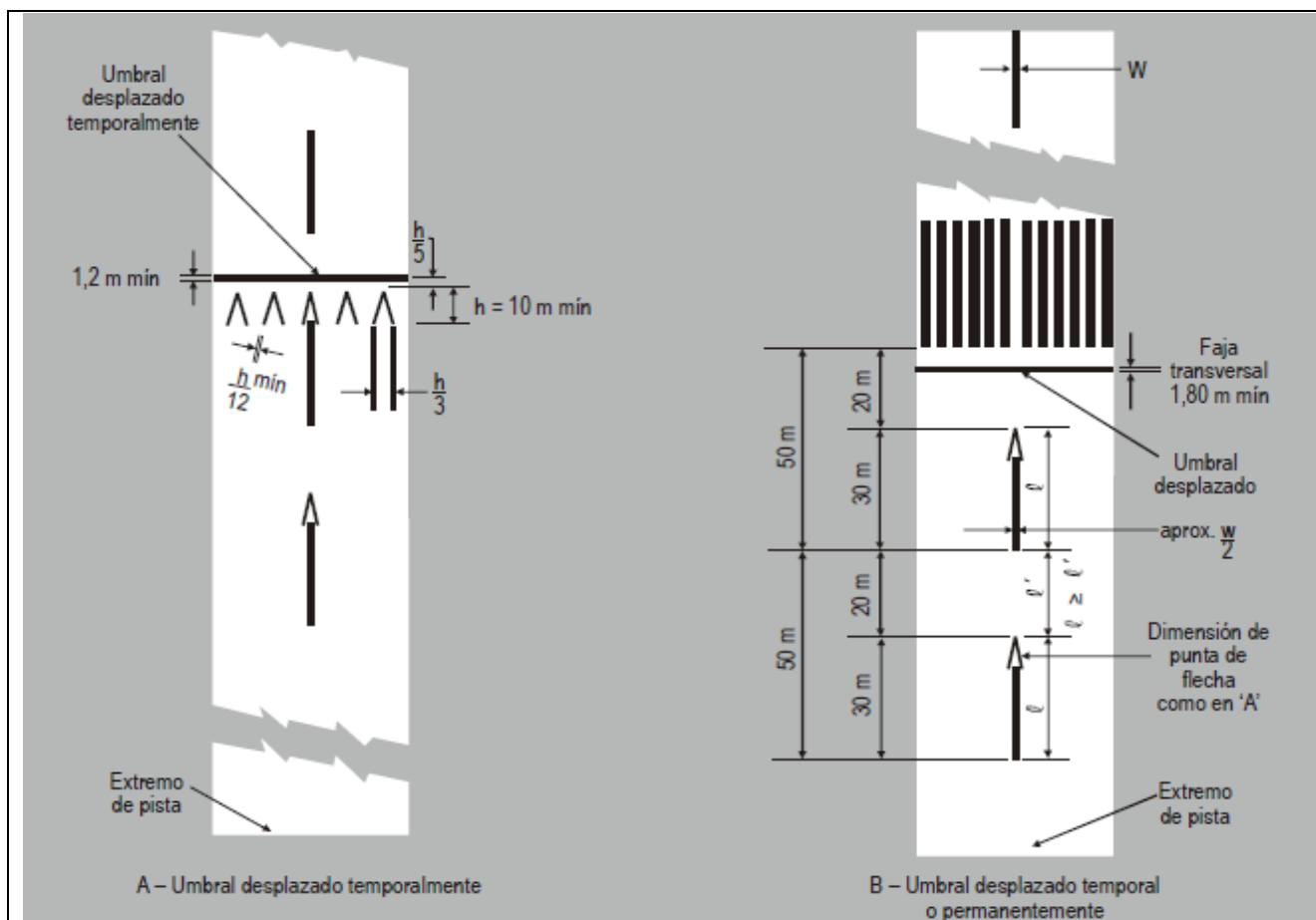
Figura E-4. Señales de umbral desplazado
