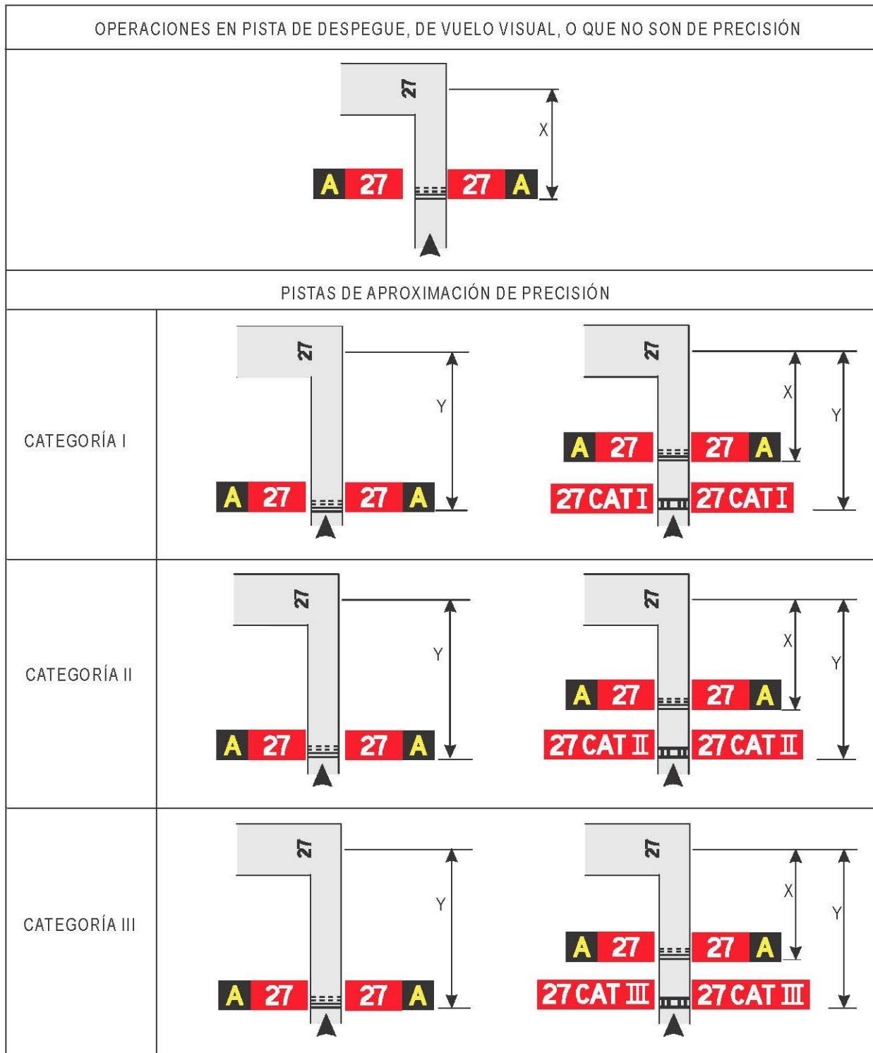
Figura E-32. Ejemplos de la ubicación de los letreros en las intersecciones de calle de rodaje/pista
