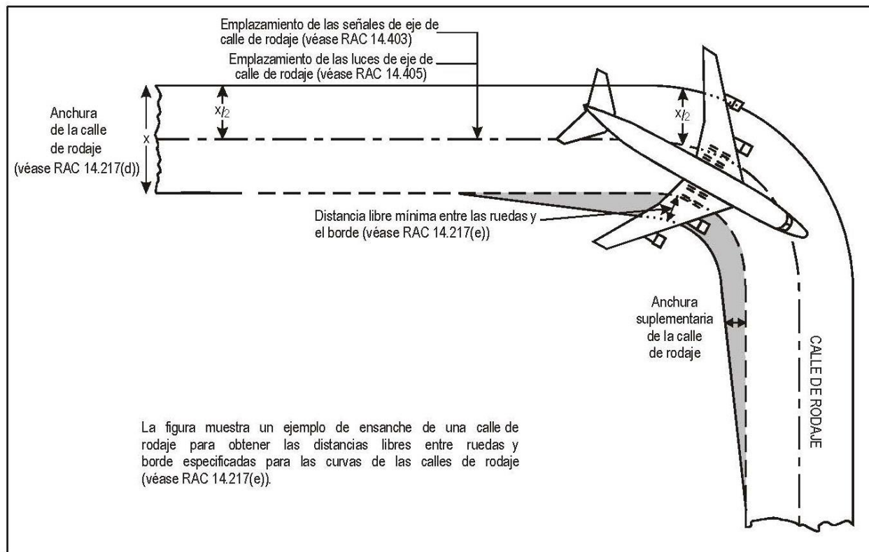
Figura C-2. Curva de calle de rodaje
