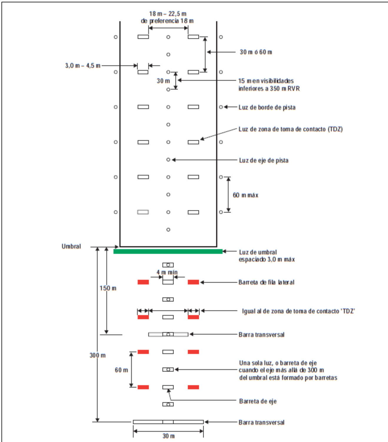
Figura E-15. Iluminación de pista y de los 300 m internos de la aproximación en las pistas para aproximaciones de precisión de Categorías II y III, cuando pueda demostrarse que se cumplen los niveles de funcionamiento de las luces especificados como objetivos de mantenimiento establecidos en la sub parte D del RAC 139
