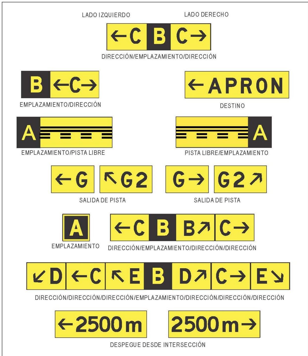
Figura E-31. Letreros de información
