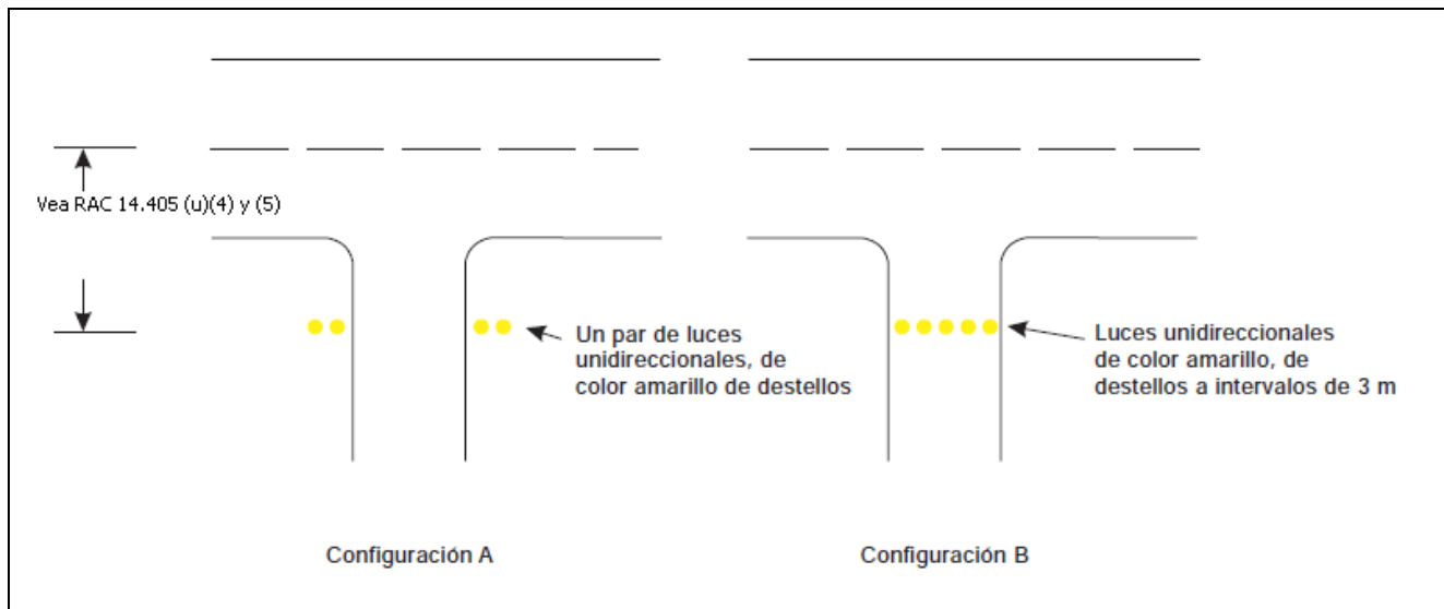
Figura E-29. Luces de protección de pista
