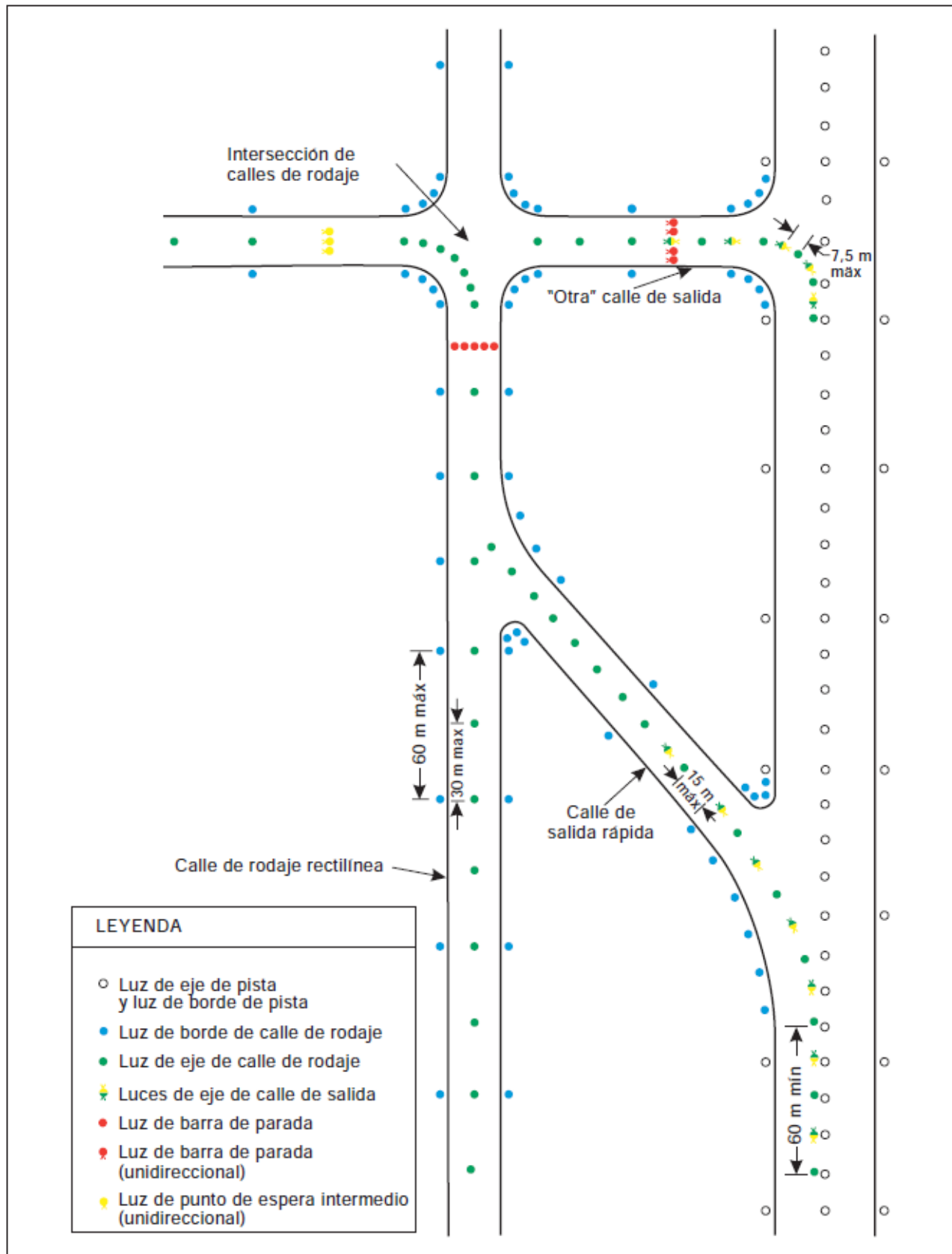
Figura E-26. Iluminación de calles de rodaje
