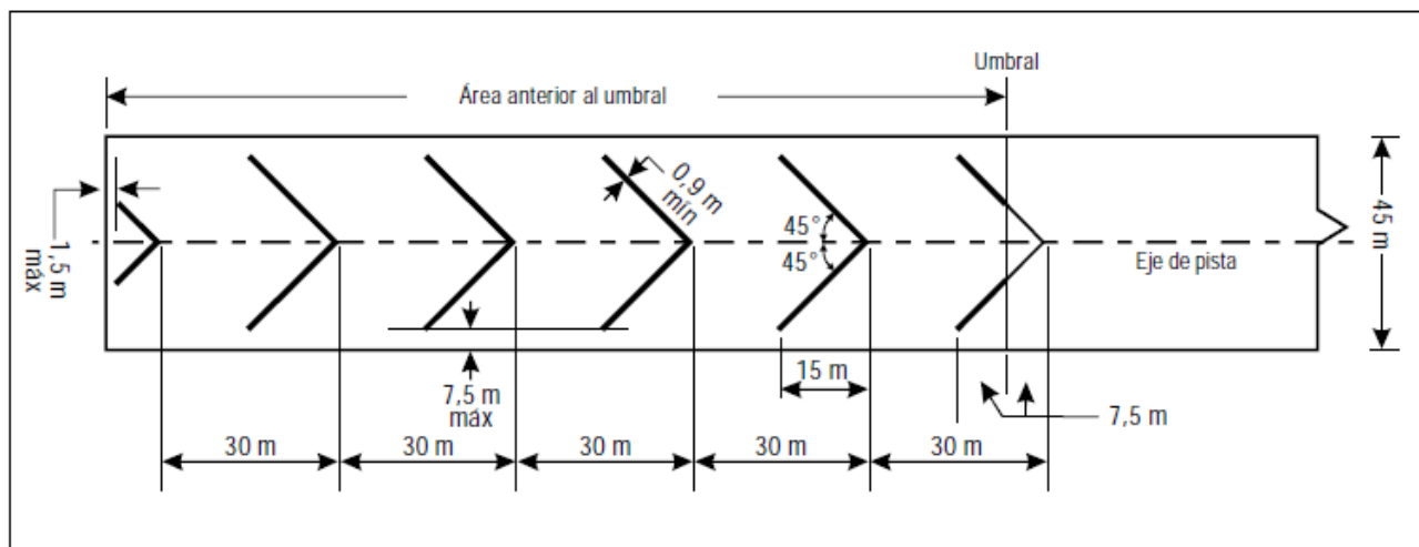
Figura G-2. Señal anterior al umbral
